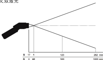
近焦距模式: 交叉双激光
