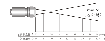
22:1 探头适用
