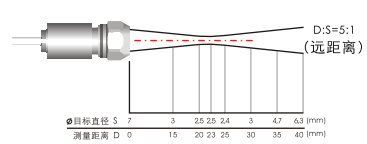
2:1 探头适用
